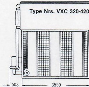
(M) Plaats van de ventilatormotor
