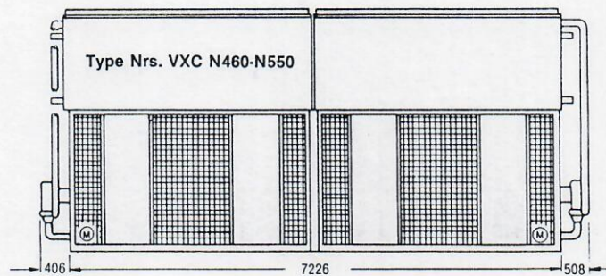
(M) Plaats van de ventilatormotor
